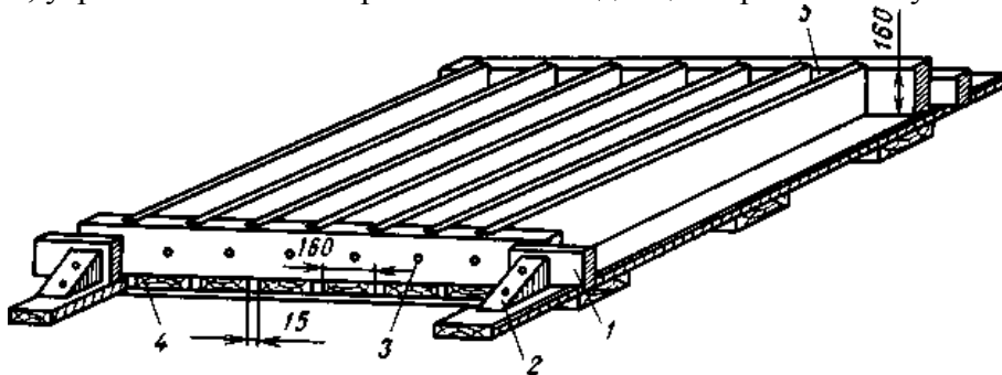
Рис. 28. Многоячейковая опалубка:
